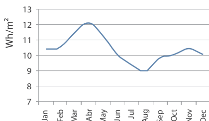
Média Irradiação Solar (Wh/m 2 )
